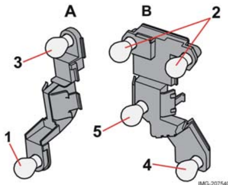
Держатель лампы
