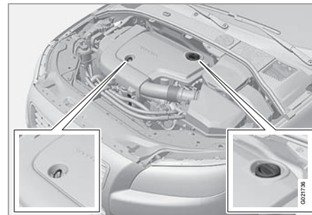
Масломерный щуп, дизельный двигатель.
