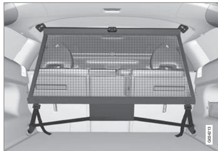
Защитная сетка крепится в четырех точках.
